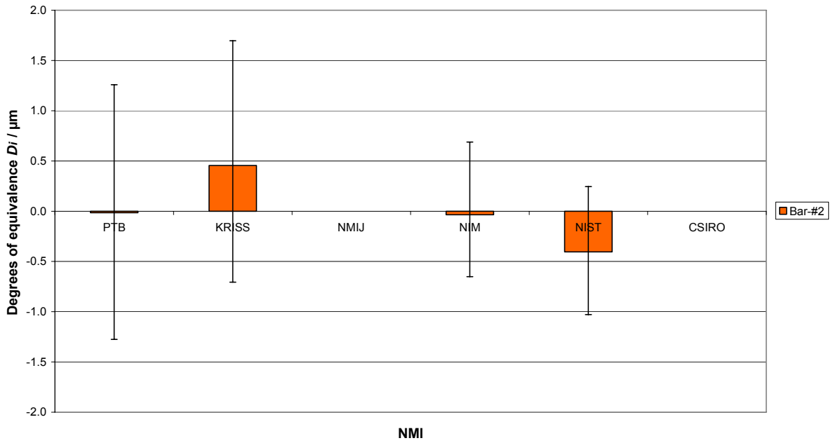
Ball Bar: 800 mm S/N UHP- 455-09
