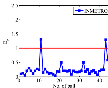
Fig. 10-30 E_n of INMETRO (Lab H8)
