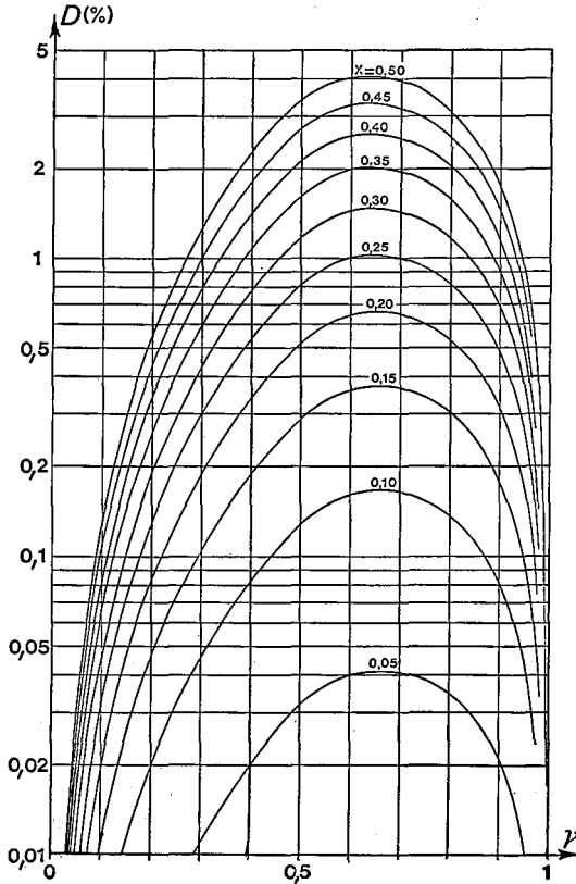
Fig. 9. — Influence D du premier temps mort cumulatif sur le taux de comptage.
