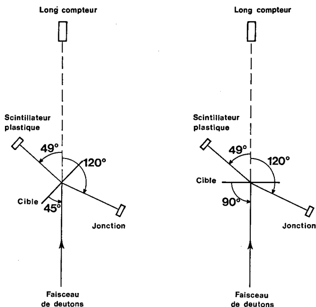
Fig. 13. — Disposition géométrique des détecteurs pour la mesure de débits de fluence.
