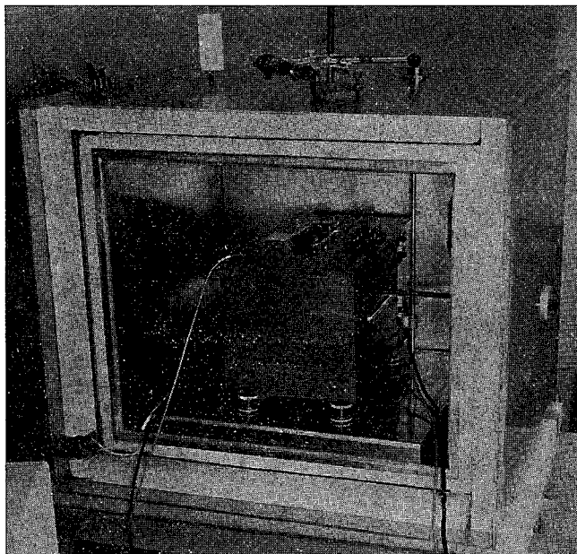
Fig. 4. — Dispositif utilisé pour modifier la température de l'air ambiant autour d'une enceinte thermorégulée transportable à 30 °C.
