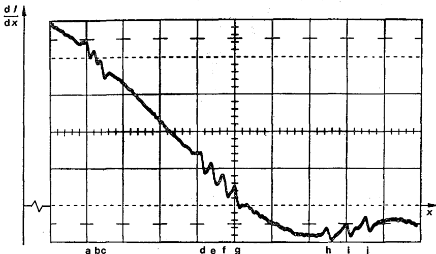
Fig. 1. — Absorption saturée de l'iode dans un laser ( \lambda = 633 \text{ nm} ).
