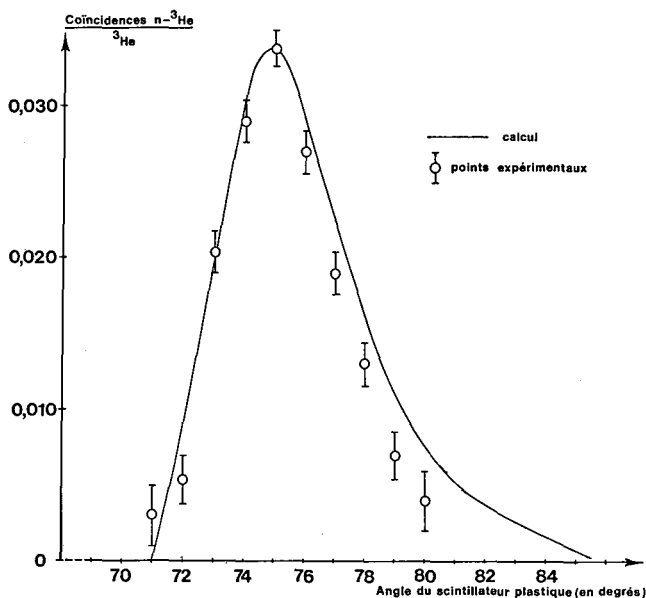
Fig. 11. — Distribution angulaire des neutrons en coïncidence avec les particules ^3\text{He} . Jonction à 90^\circ ; énergie des deutons incidents: 100 keV.
