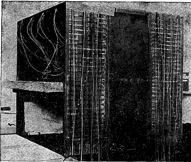
Fig. 5. — Chambre intérieure en cuivre de l'enceinte thermorégulée du B.I.P.M., sur les parois de laquelle sont collées les plaquettes constituant les « shunts thermiques. »
