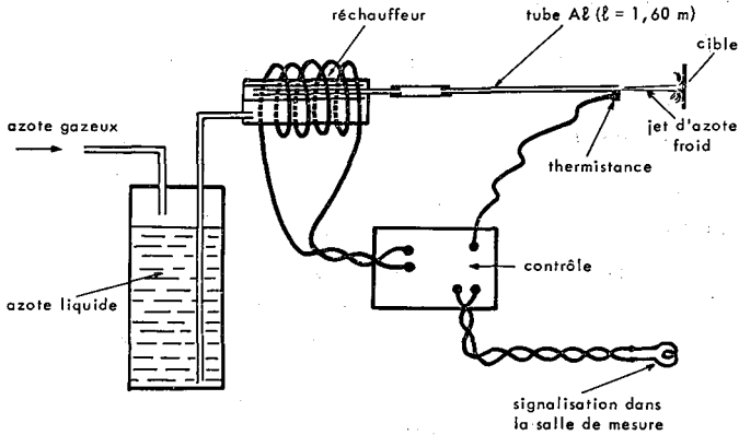
Fig. 12. — Système de refroidissement de la cible.
