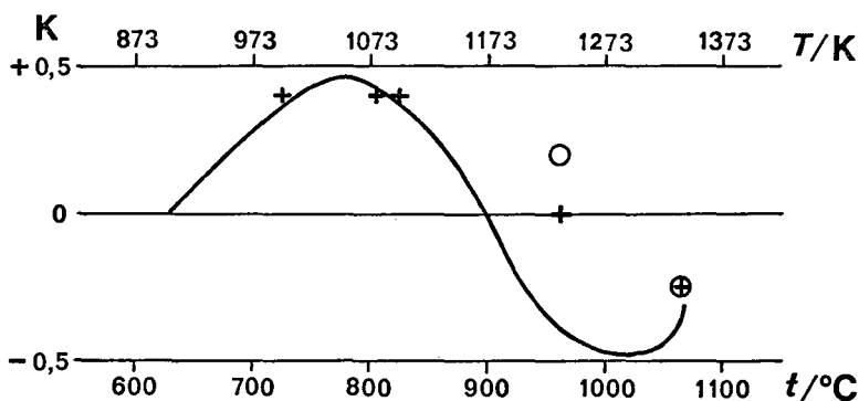
Fig. 3. — Différence Échelle thermodynamique — E.I.P.T.-68. Température de référence 630,74 °C; c_2 = 0,014\ 388\ \text{m} \cdot \text{K} .
