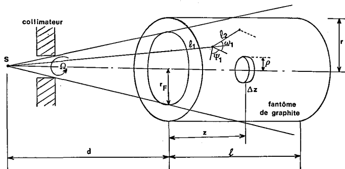
Fig. 6. — Schéma de principe pour le calcul de la fluence des photons à l'intérieur d'un fantôme de graphite.
